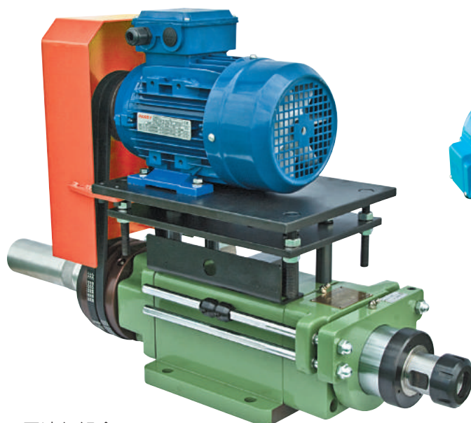
馬達架組合
