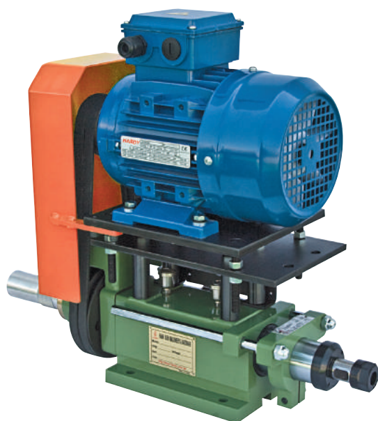
馬達架組合
